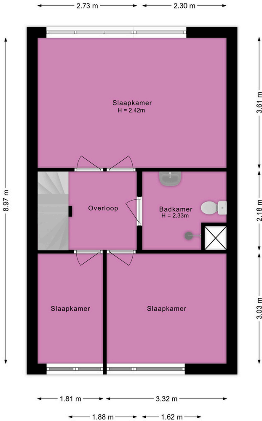
Zinniadal 13 Leiden 1e Verdieping
