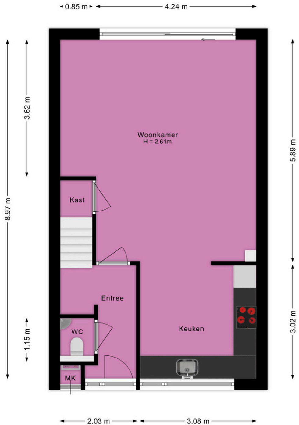
Zinniadal 13 Leiden Begane grond
